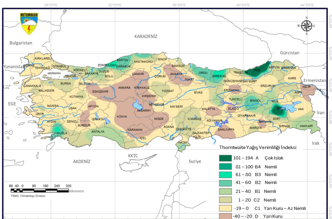
Grafik 4: Türkiye İklim Sınıflandırması
