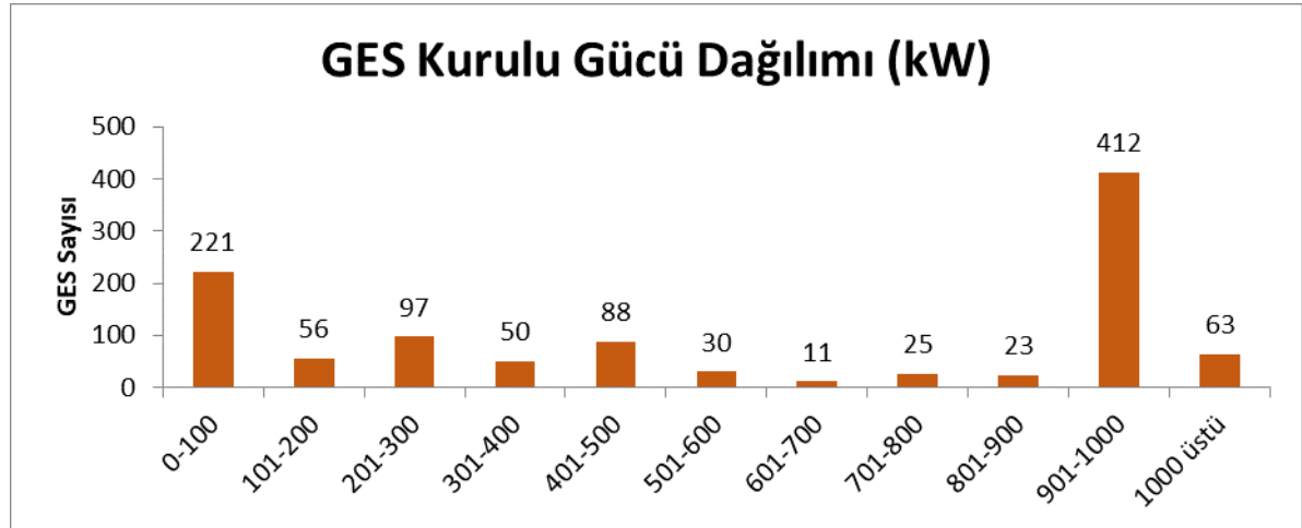
Grafik 8: Kurulu Güç Bazında GES'lerin Dağılımı
